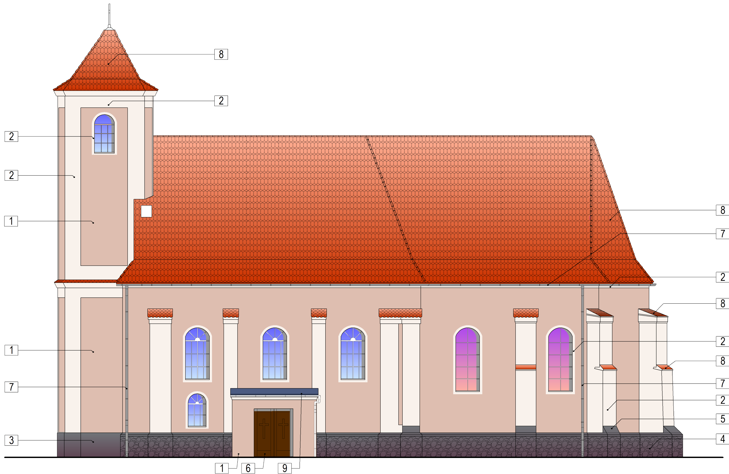
ELEVACJA POŁUDNIOWA
